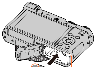
Рычажок отжимания
